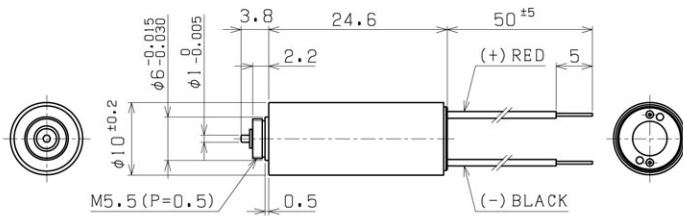
※ケーブル位置は参考です THE CABLE LOCATION IS FOR REFERENCE ONLY. Unit : mm
